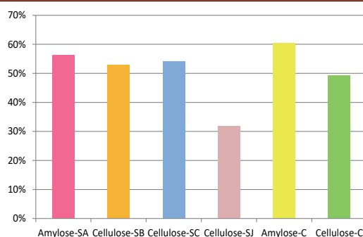
キラル分離用カラムのスクリーニングヒット率
