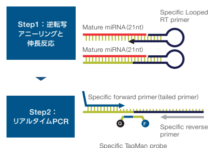
図 1. TaqMan MicroRNA Assay のワークフロー
