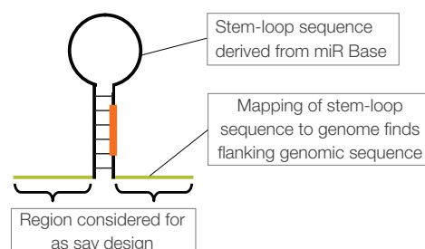
図 2. TaqMan Pri-miRNA Assay のデザインアプローチ
